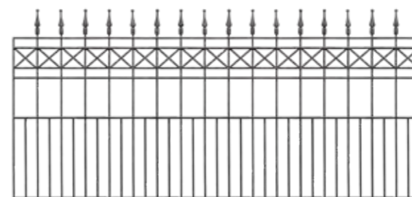
MAILAND mit Kreuz-Ornamenten und Zierspitzen Seite 48
