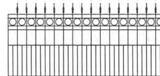
FLORENZ mit Kreis-Ornamenten und Zierspitzen Seite 46
